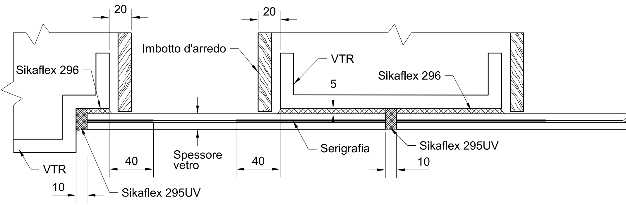
DETTAGLIO INCOLLAGGIO VETRI E SERIGRAFIA SCALA 1:2
