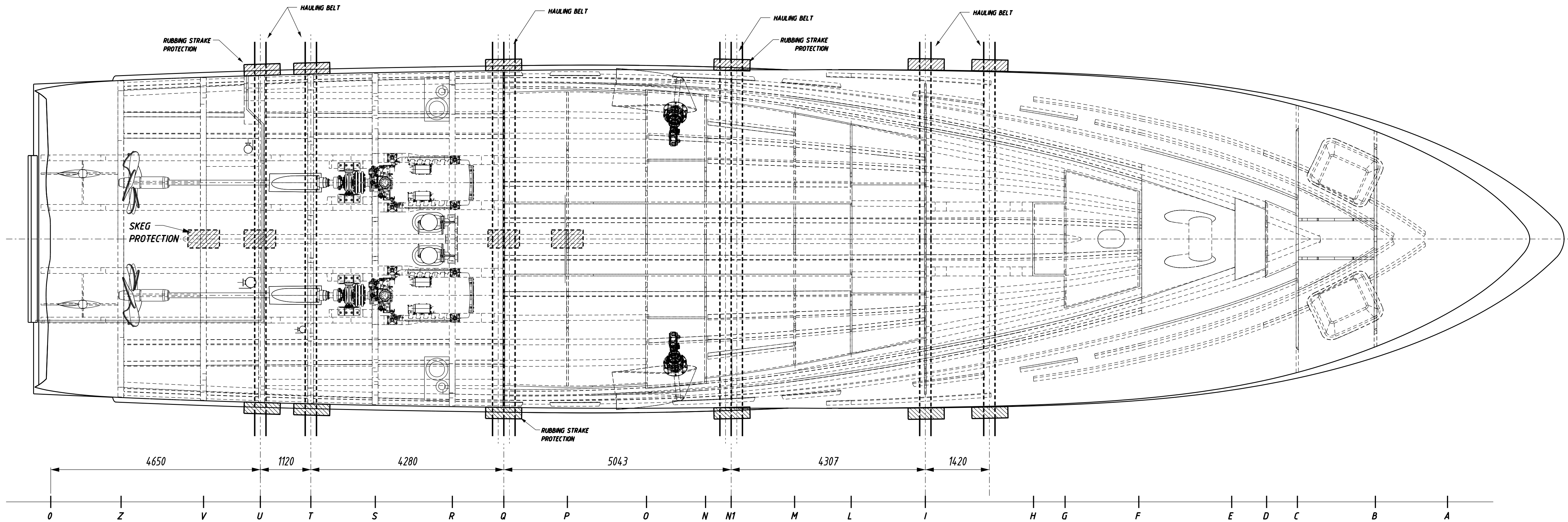
PIANTA POSIZIONAMENTO FASCE PER ALAGGIO HAULING BELT PLAN POSITIONING
